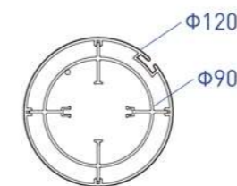
二重生地巻き取りパイプ 断面図
