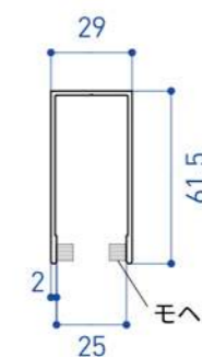
遮光ガイドレール 断面図
