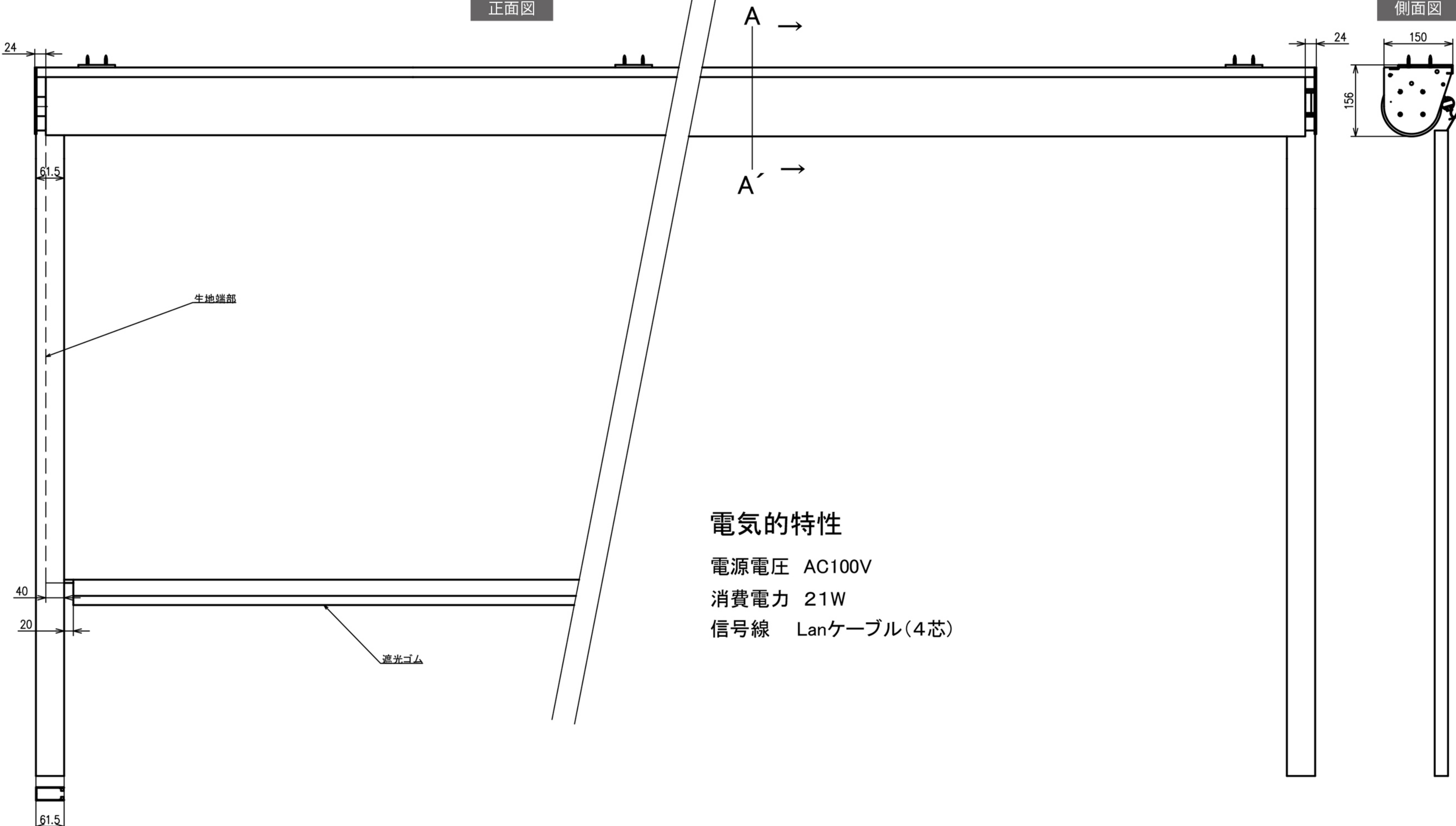
正面図
